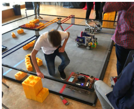
Twee robots in actie op het officiële speelveld van de First Tech Challenge
